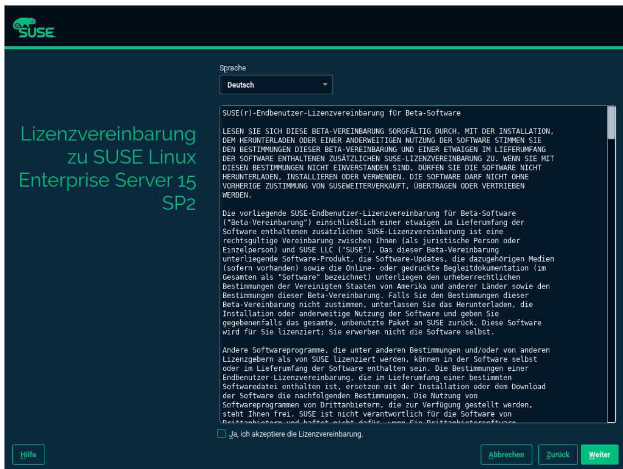
ABBILDUNG 8.2: LIZENZVEREINBARUNG
