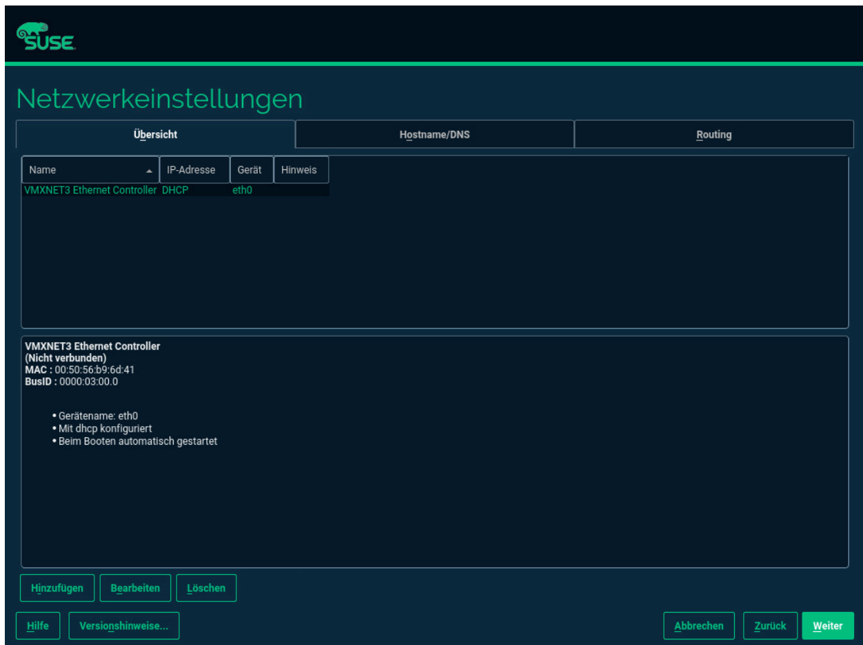
ABBILDUNG 8.5: NETZWERKEINSTELLUNGEN
