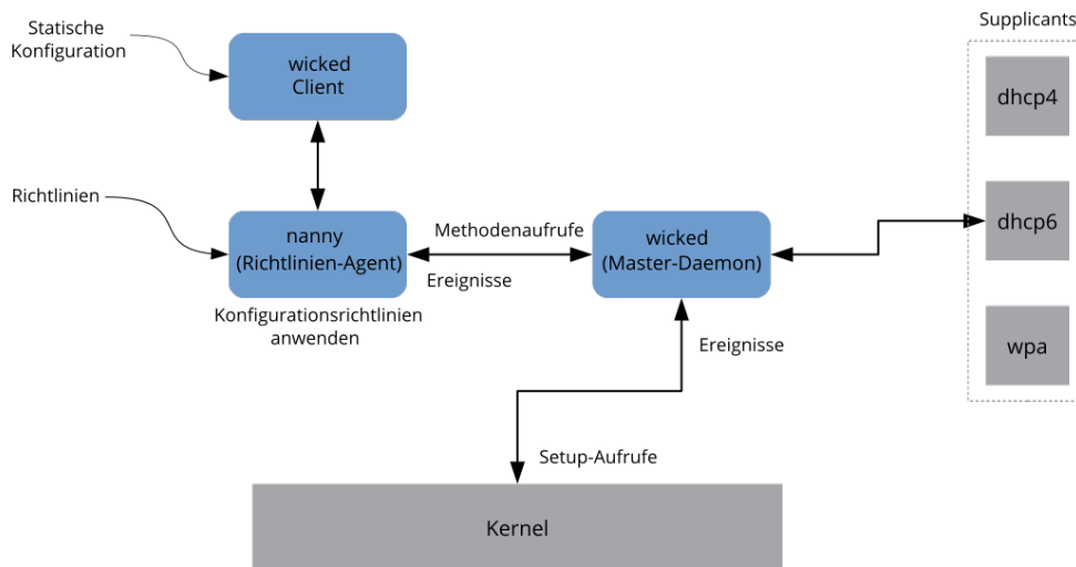
ABBILDUNG 23.4: wicked-ARCHITEKTUR
