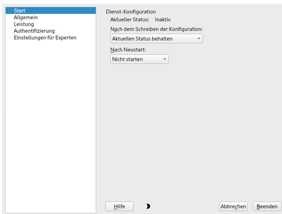
ABBILDUNG 43.1: FTP-SERVERKONFIGURATION – START
