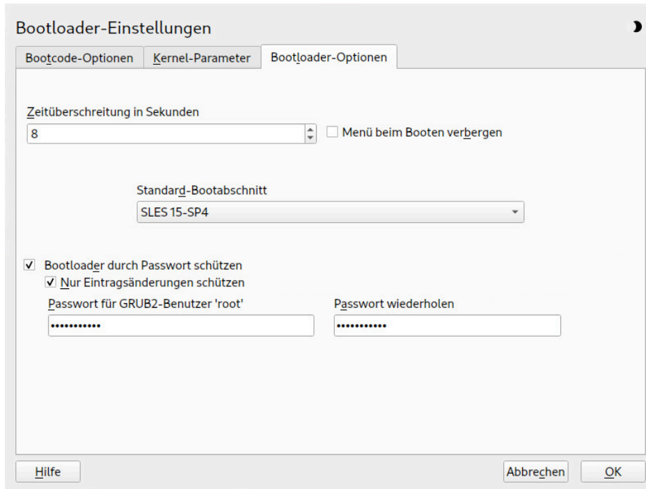
ABBILDUNG 18.3: BOOTLOADER-OPTIONEN
