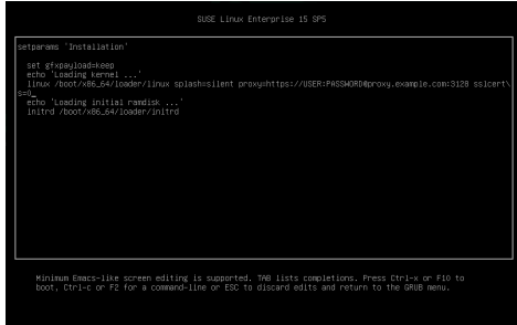
FIGURA 7.3: EDITOR DE OPÇÕES DO GRUB
