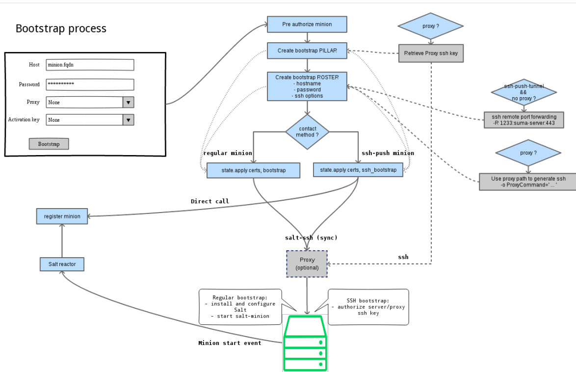
图表 1. Salt SSH Bootstrap Process
