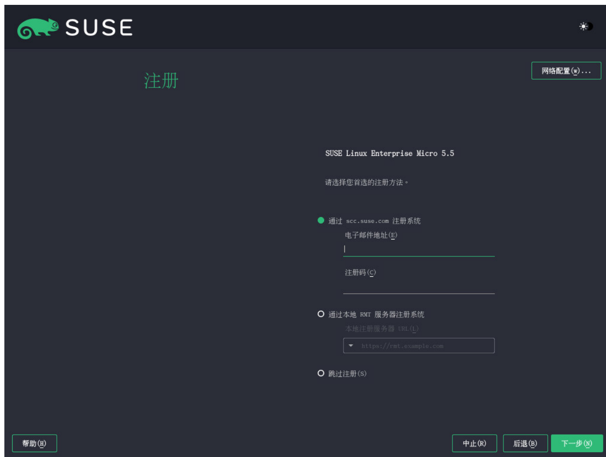
图 12.6：注册
