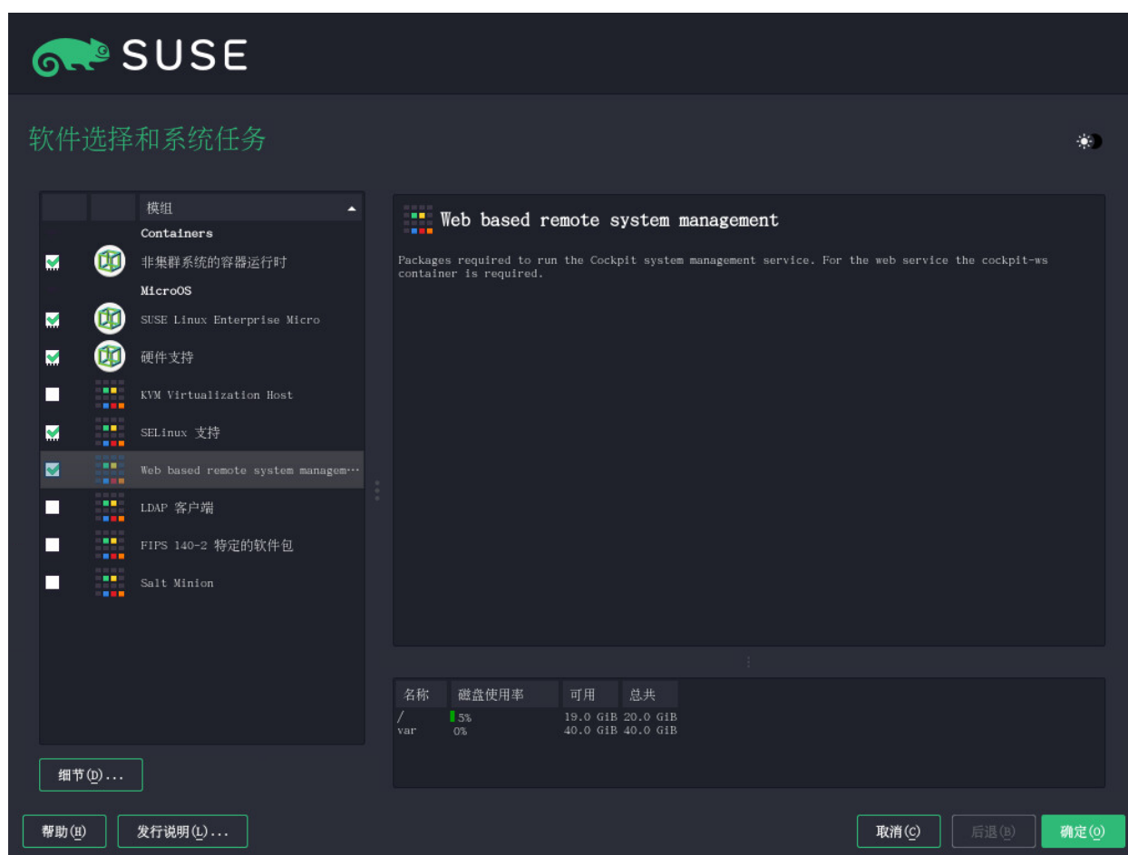
图 12.13：软件配置
