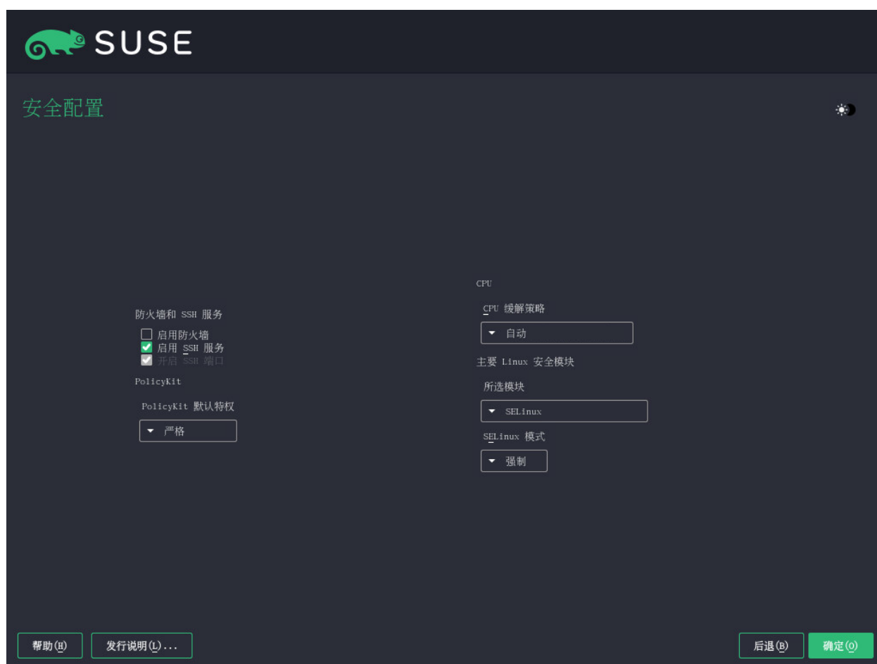
图 12.18：安全配置
