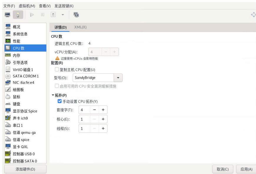
图 14.6：处理器视图
