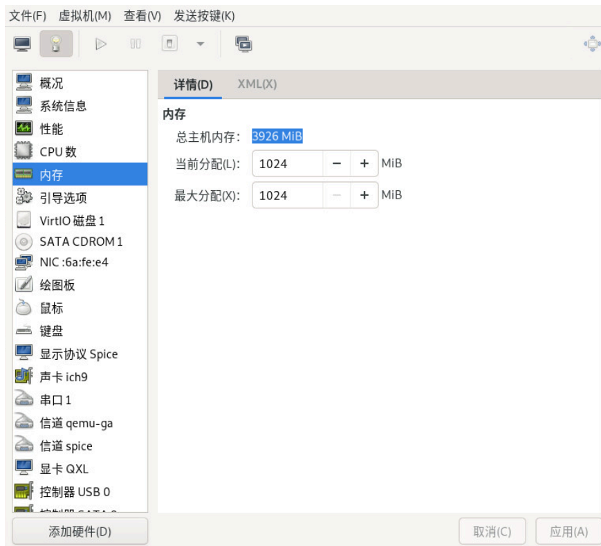
图 14.7：内存视图
