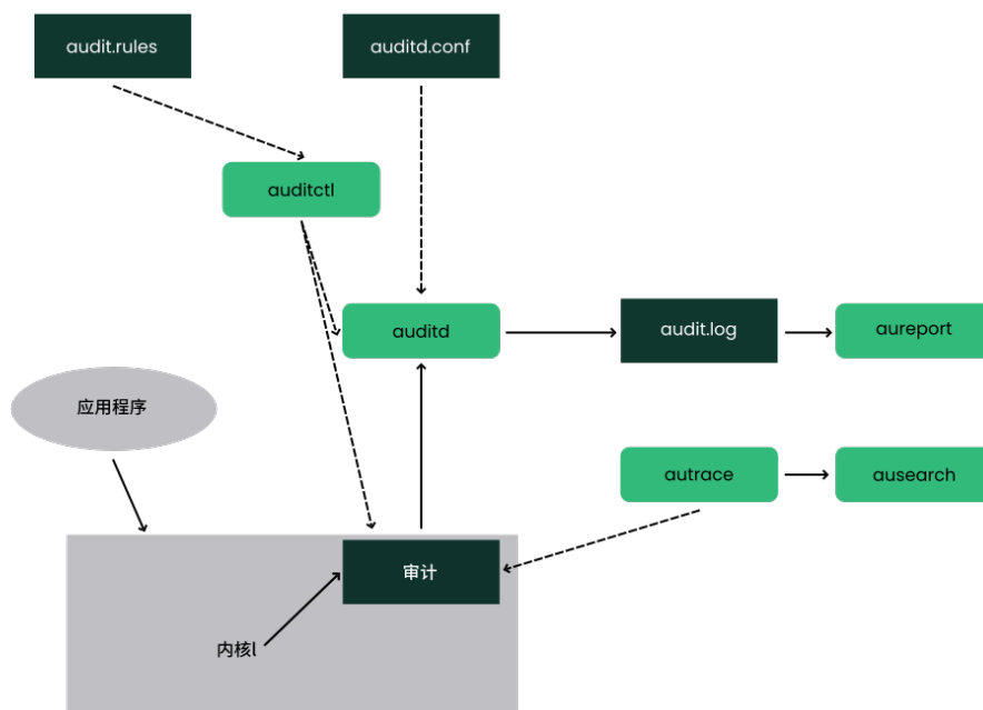
图 44.1：Linux 审计组件简介
