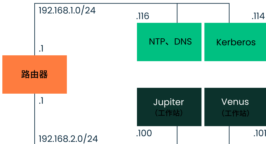
图 6.1：KERBEROS 网络拓扑
