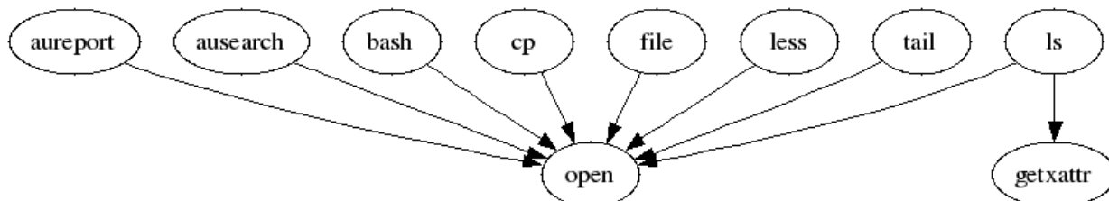
图 44.2：流程图 — 程序与系统调用之间的关系
