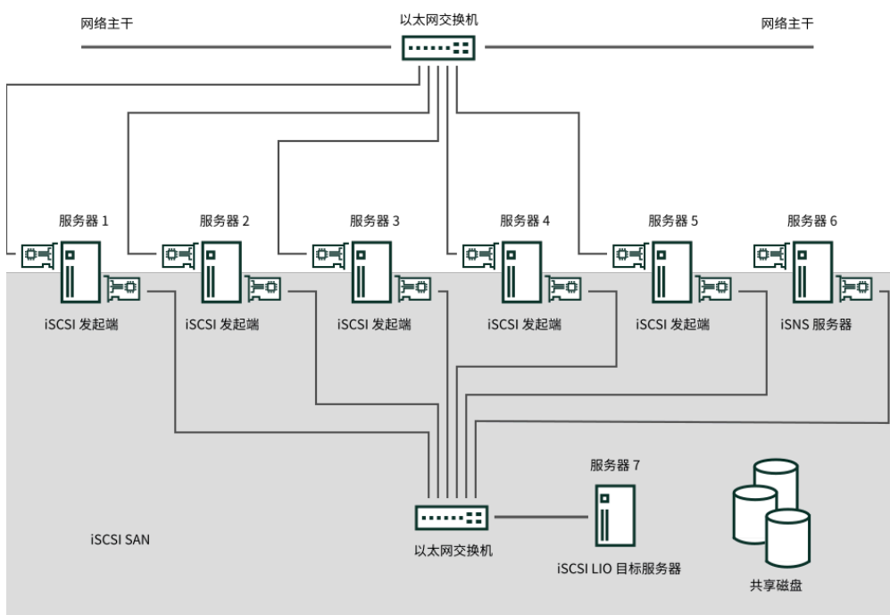
图 15.1：使用 iSNS 服务器的 iSCSI SAN
