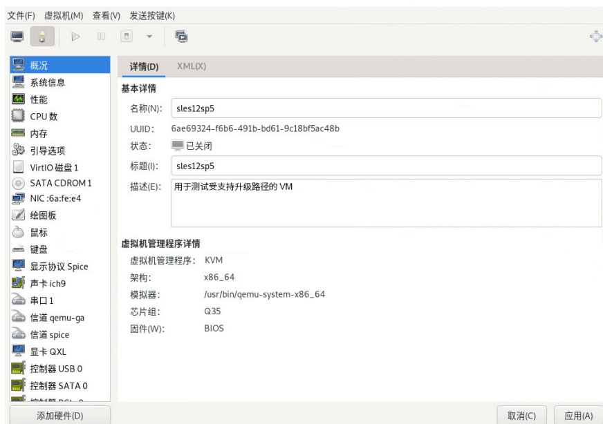
图 14.2：概览细节
