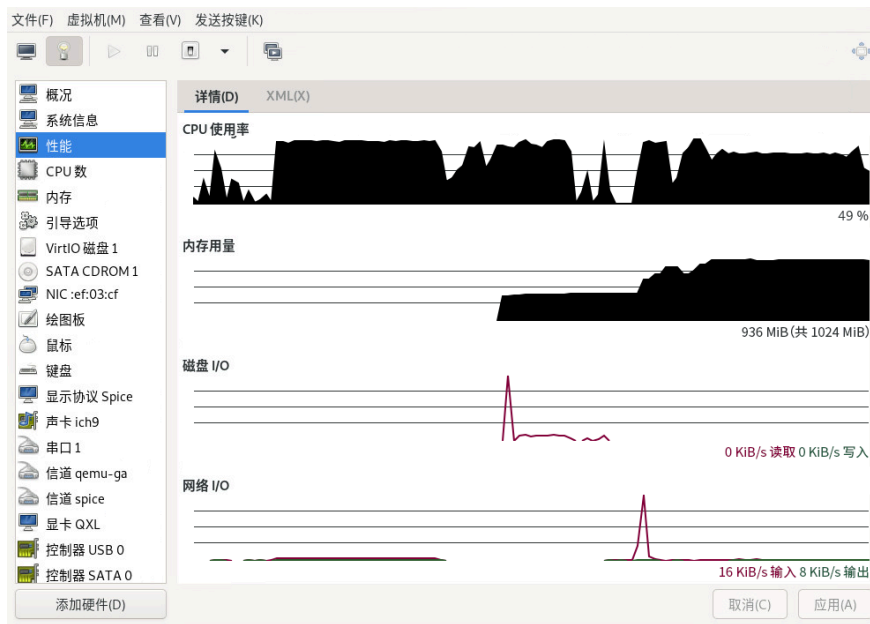
图 14.4：性能
