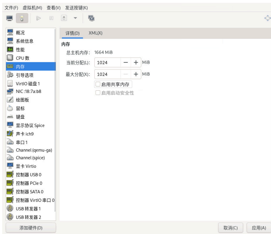
图 14.7：内存视图
