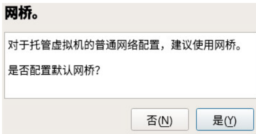
图 33.2：网桥
