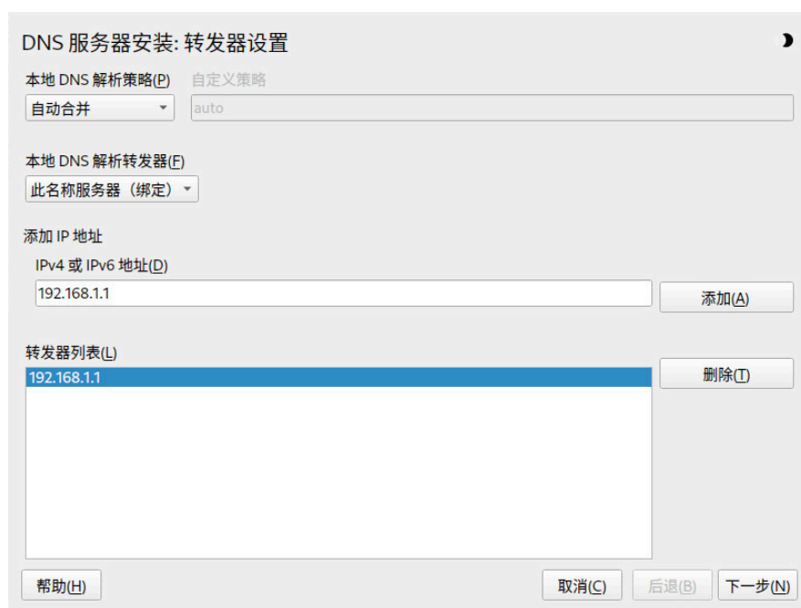
图 39.1：DNS 服务器安装：转发器设置
