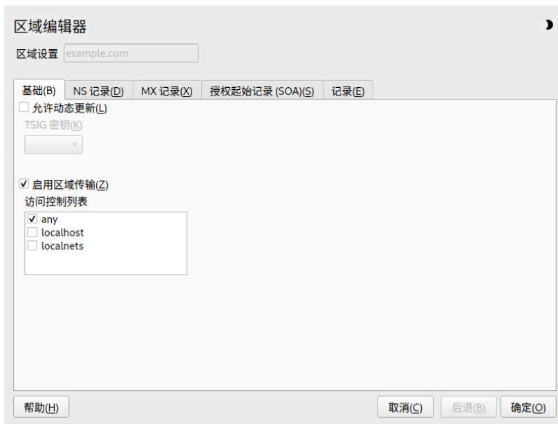
图 39.5 : DNS 服务器：区域编辑器（基本）
