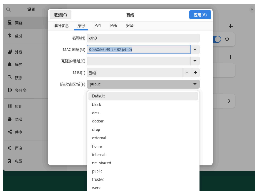
图 31.2：NETWORKMANAGER 中的 firewalld 区域
