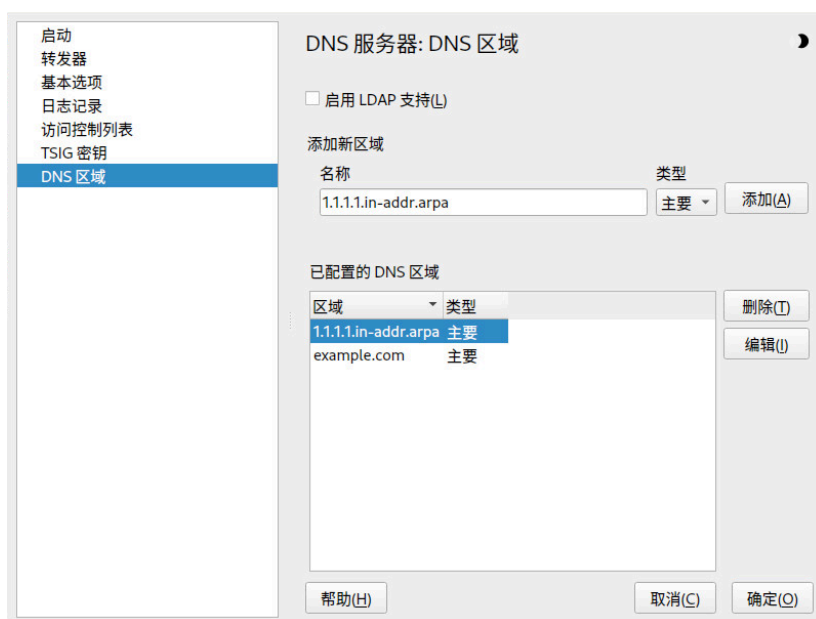
图 39.10：添加反向区域
