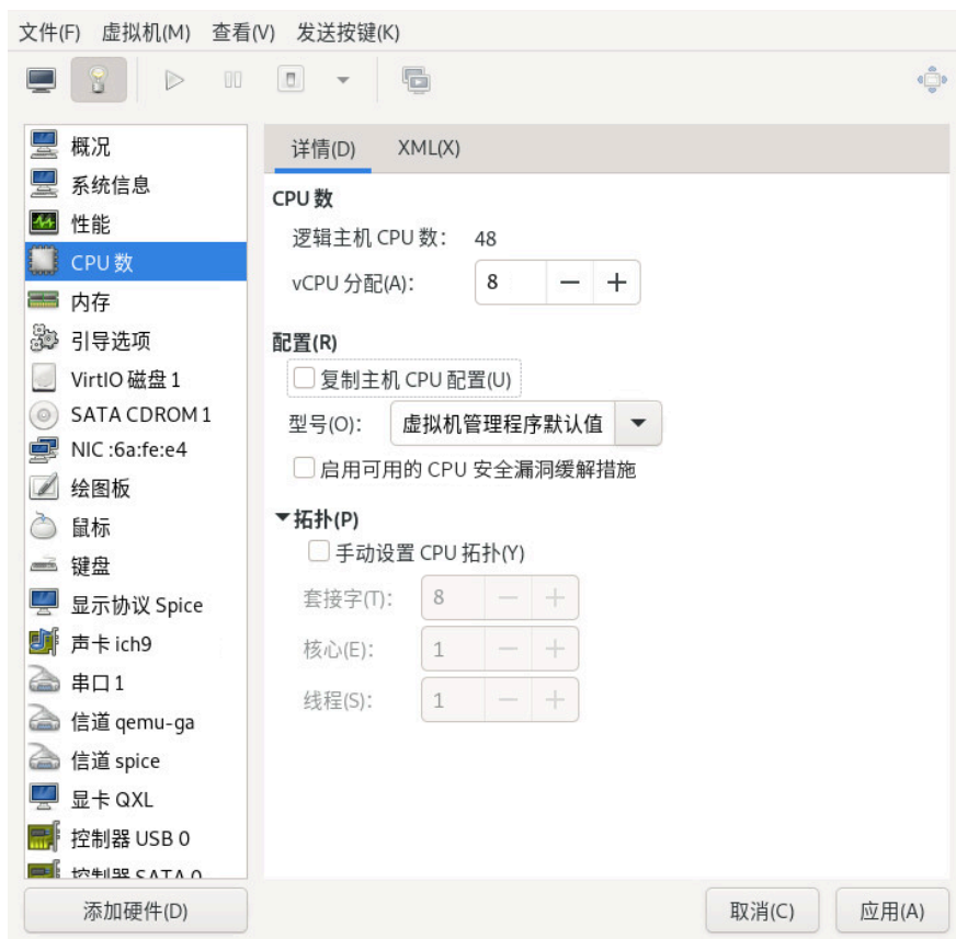
图 14.6：处理器视图
